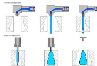
Figura No. 21 Proceso extrusión soplado
